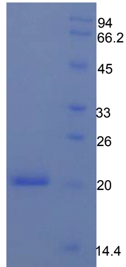
15% SDS-PAGE
